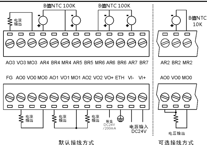
LS21-E4DA4N(R) 端子接线方式
