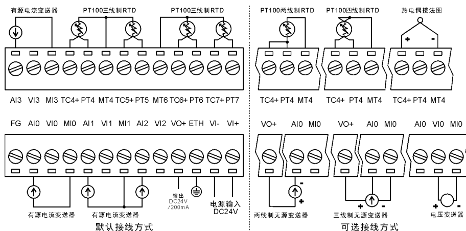
LS21-E4AD4P(T)端子接线方式
