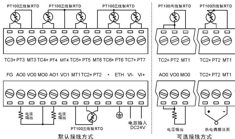
LS21-E2DA6P(T) 端子接线方式
