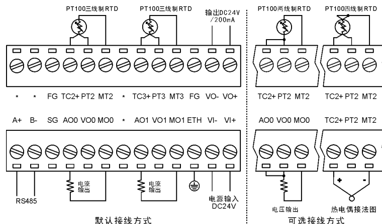
LS21-E2DA2P(T) 端子接线方式
