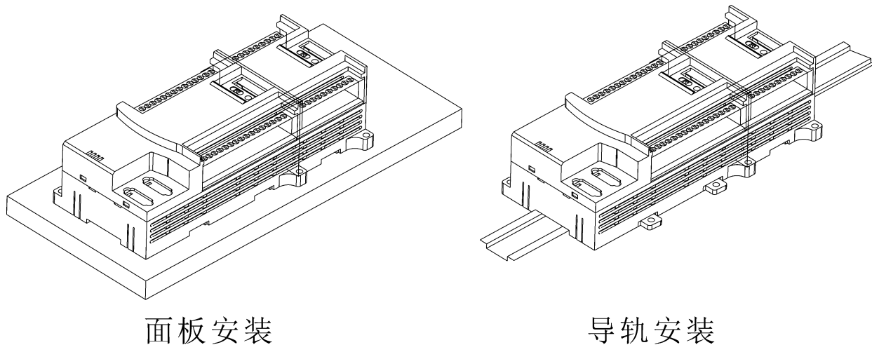
图 1.4.4 LS 系列 PLC 的安装方式
