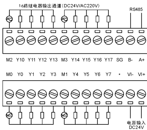
LS21-E16YR端子接线方式
