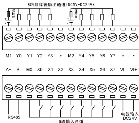
LS21-E8X8YT端子接线方式
