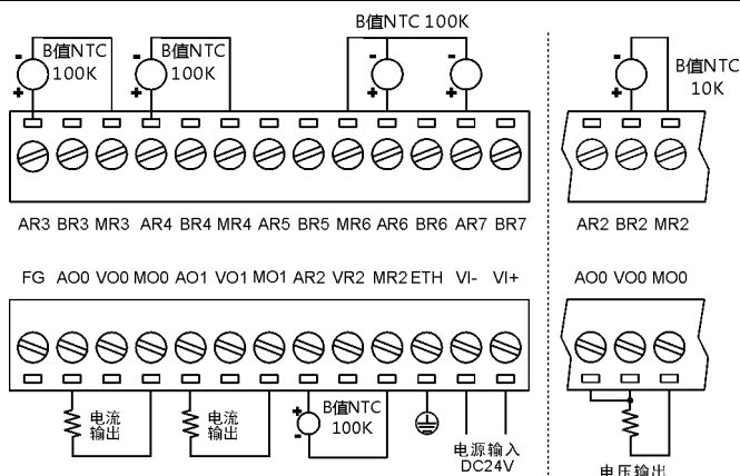
默认接线方式 LS21-E2DA6N(R) 端子接线方式
