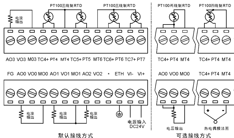
LS21-E4DA4P(T)端子接线方式
