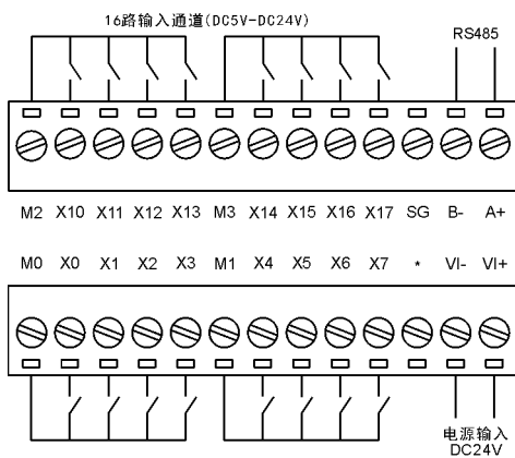
LS21-E16X端子接线方式
